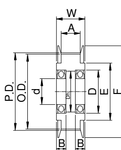
兩側軸承型
