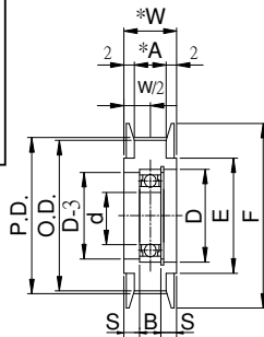
中心軸承型
