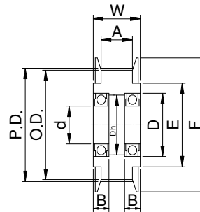
兩側軸承型
