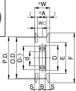
▲S8M型 (中心軸承型)
