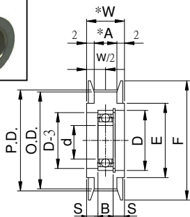
▲S2M型 (中心軸承型)
