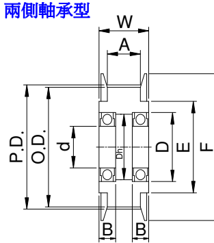
兩側軸承型
