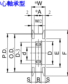
中心軸承型
