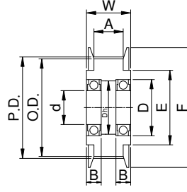
兩側軸承型
