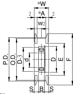
中心軸承型
