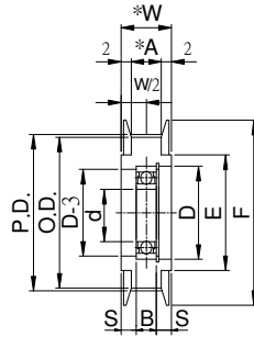
中心軸承型
