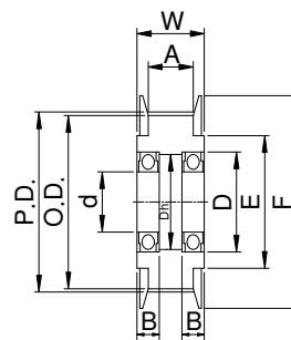
兩側軸承型
