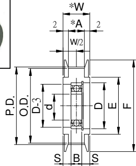
中心軸承型
