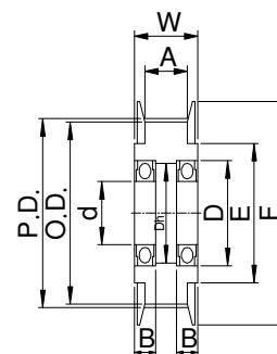
兩側軸承型
