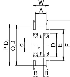
兩側軸承型
