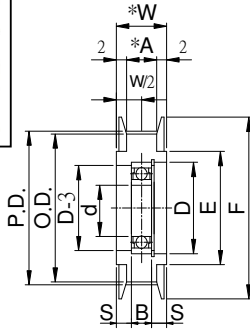
中心軸承型
