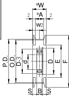
中心軸承型
