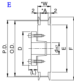
皮帶輪形狀：
